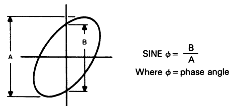
Fig. 25 Phase shift calculation
