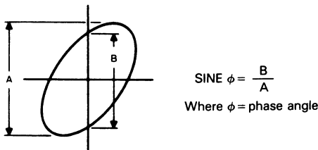
Fig. 25 Phase shift calculation
